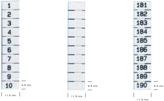
DY 10/6.5 TYP / TYPE DB 10/6.5 TYP / TYPE DO 10/6.5 TYP / TYPE
